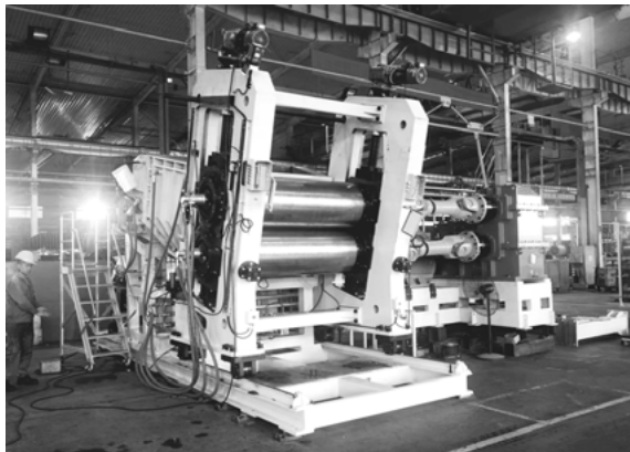
图2 580锥形双螺杆挤出压片机
