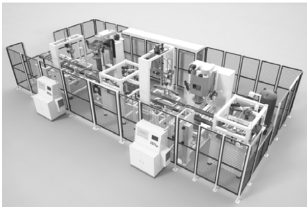
图1 PUB-3轿车轮胎均匀性/动平衡联机检测线
